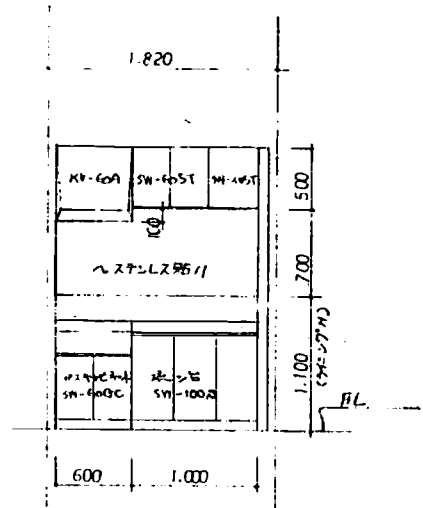
洗面台 1/50
